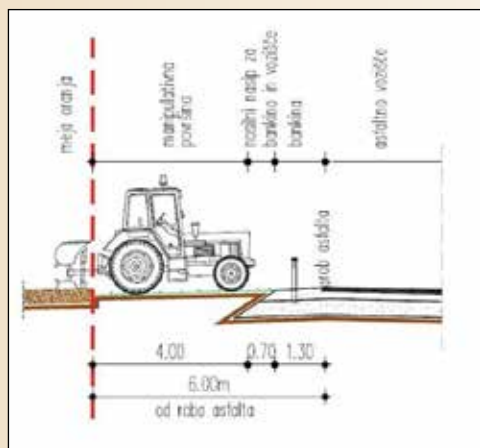
Oranje pravokotno na cesto
